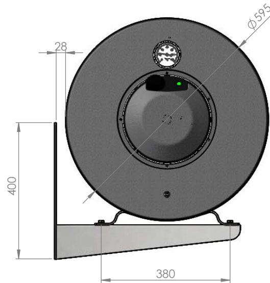
Instalace bojleru o průměru nádoby 480mm
